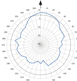
5000-6000 MHz
