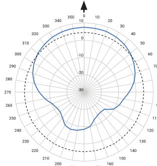
600-900 MHz
