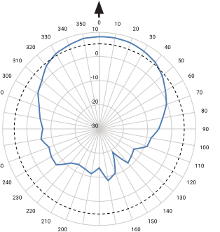
1700-2700 MHz
