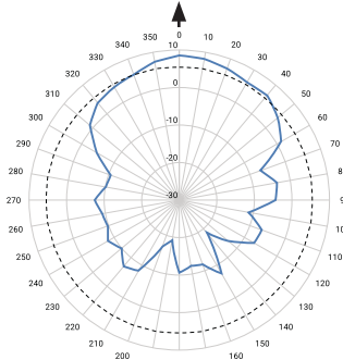
3500-4200 MHz
